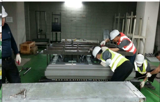
정류기용 변압기 코어조립 2
