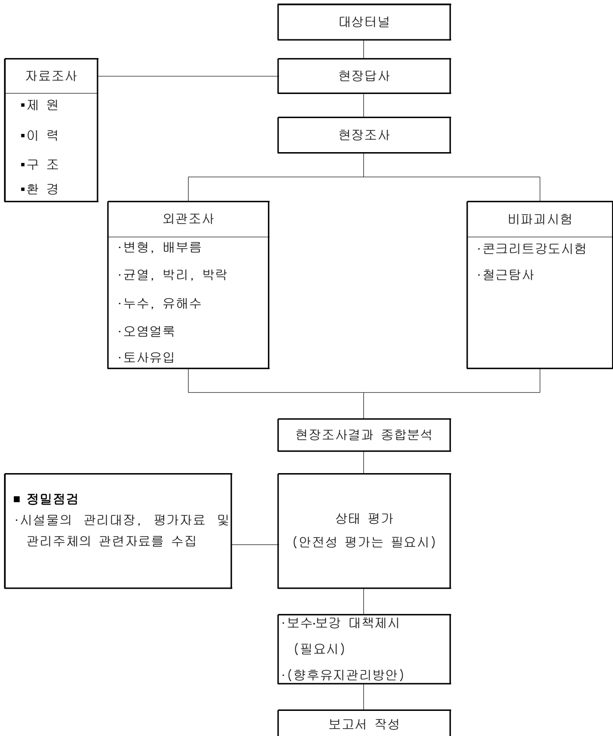
【그림 1-1】 정밀점검 수행 흐름도
