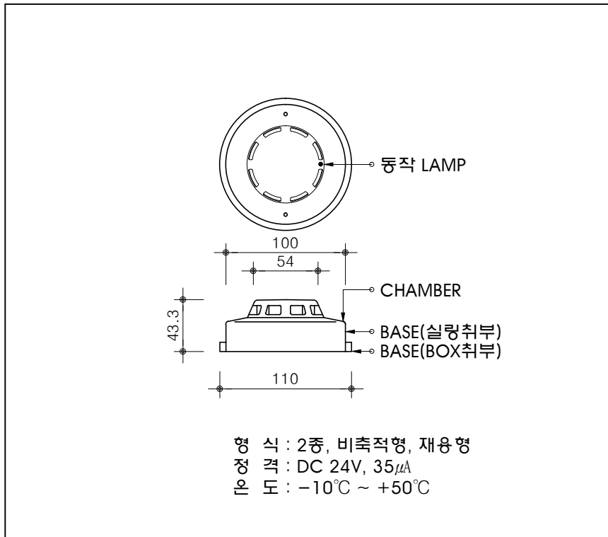
연기 감지기 (광전식)
