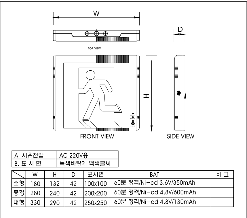
고휘도 피난구 유도등 (LED)
