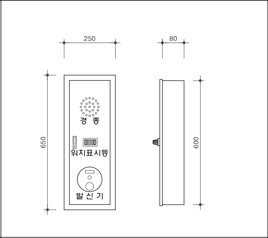
수동 발신기 (단독형)
