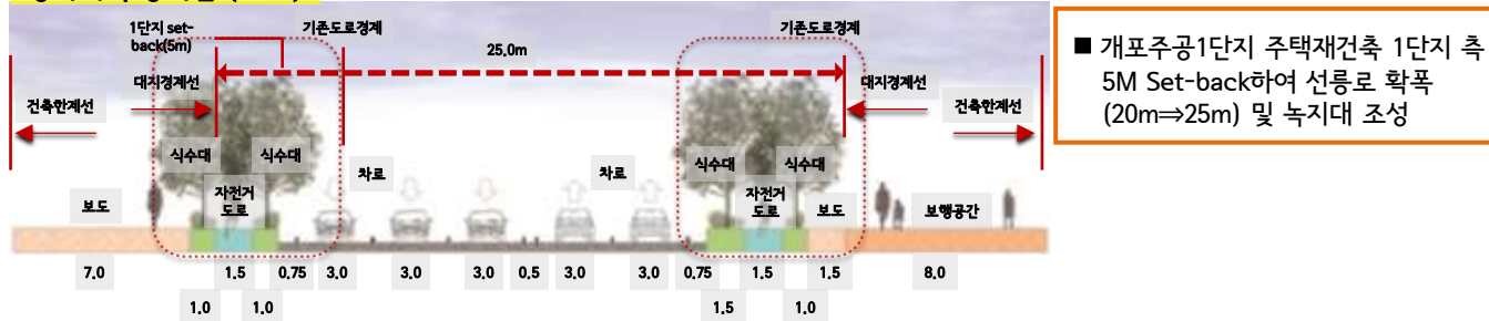
정비계획 장기안 (B-B')
