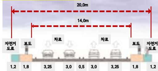
선릉로 현황단면 (B-B')
