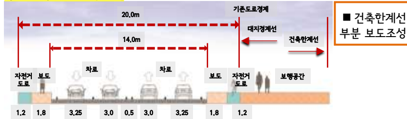
정비계획 장기안 (B-B')
