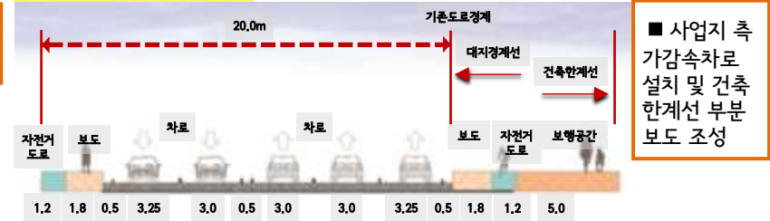
정비계획 단기안 (b-b')
