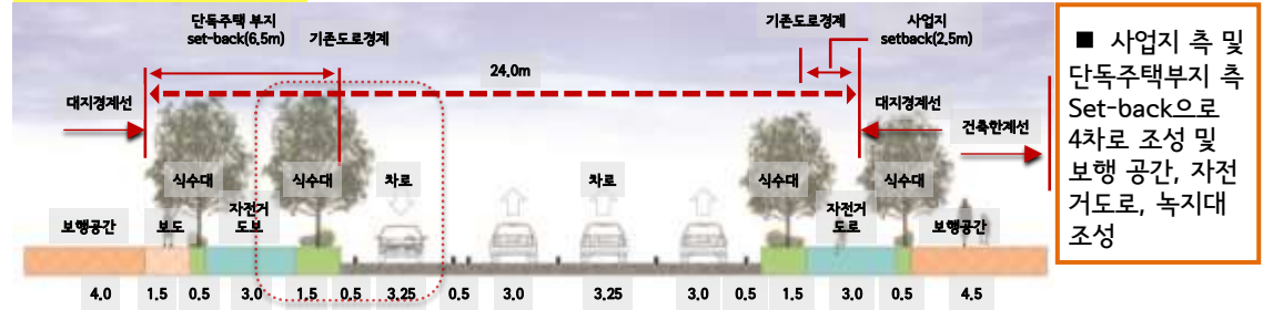
정비계획 장기안 (A-A')
