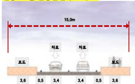
선릉로4길 현황단면 (A-A')
