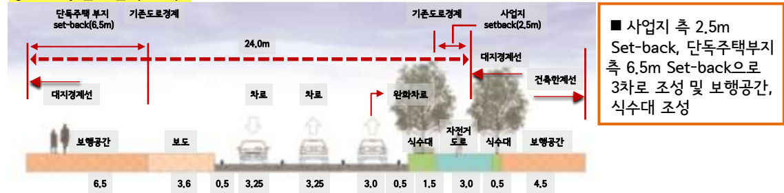
정비계획 단기안 (A-A')
