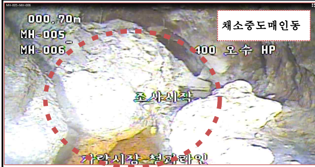
CCTV 조사 : 채소중도매인동 (하단부 관로파손 - 하부 세굴층)
