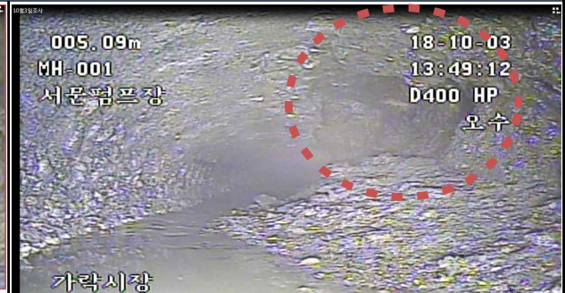
CCTV 조사 : 수산동 가압펌프장 (상단부 관로파손 - 열화부식 콘크리트 탈락)
