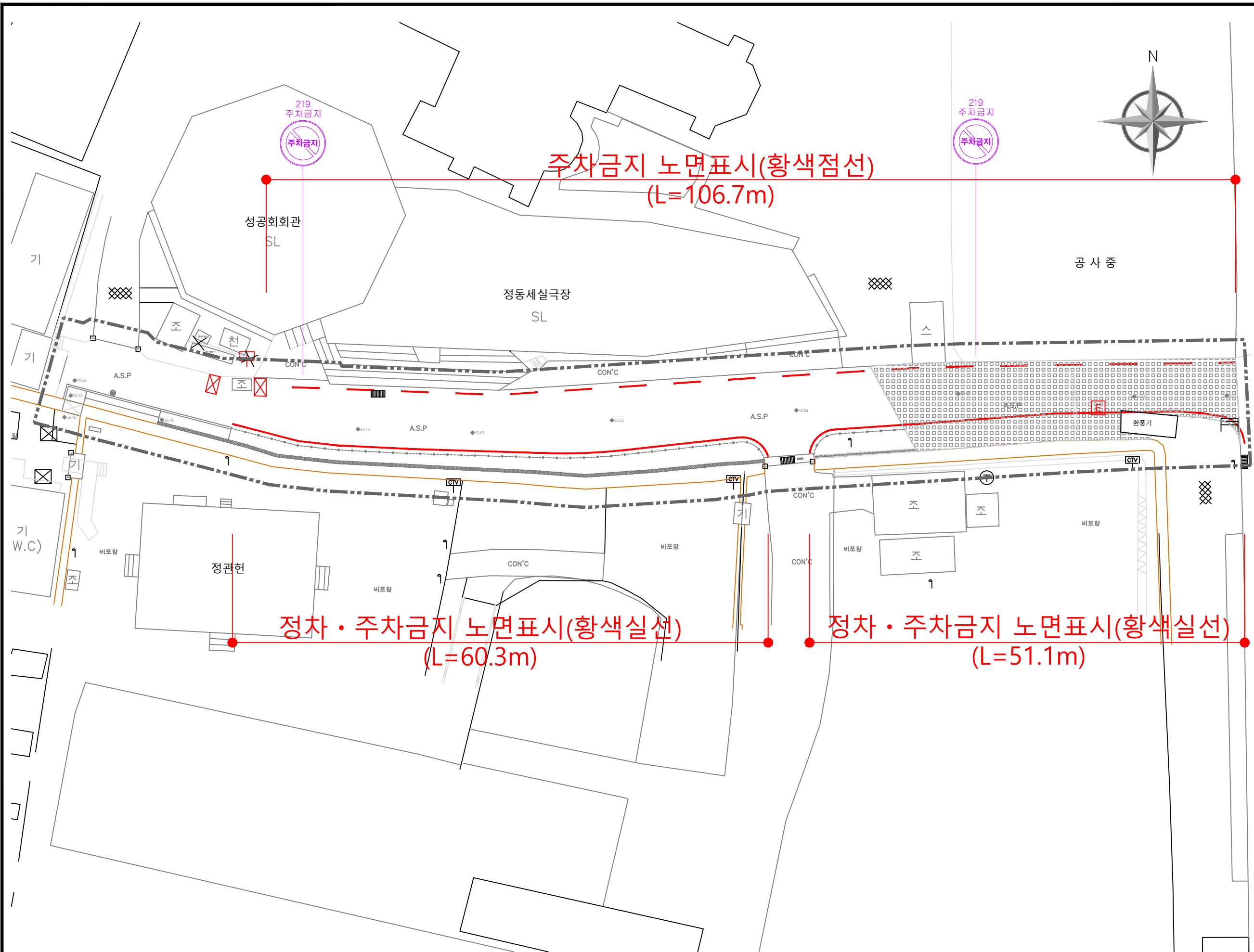
1 공사계획평면도 축척 : 1 / 200(A3:1/400)
