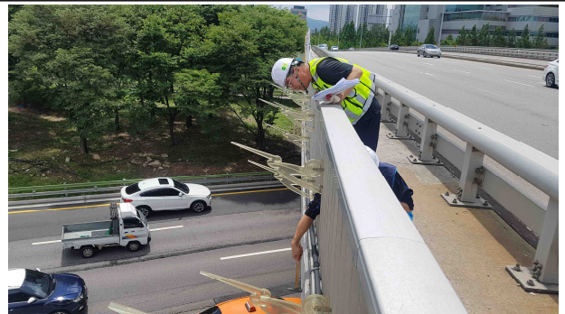
공 사 명 : 2016 한강교량 일상유지 보수공사 공사내용 : P18~P20 콘크리트 단면보수 점검결과 : 보수상태 양호
