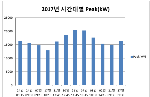
<동절기 가락시장 시간대별 전력 Peak>
