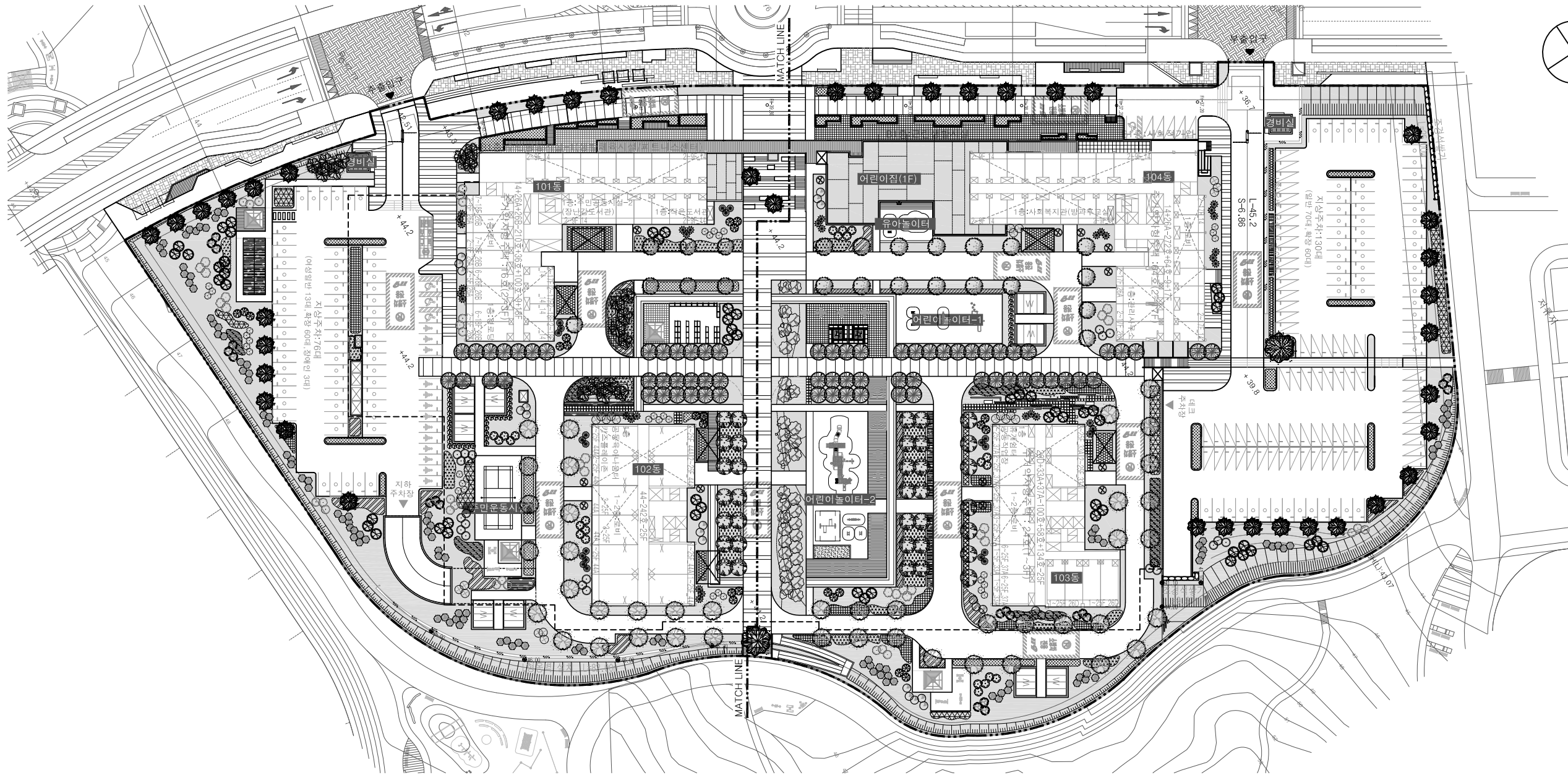
1 식재계획도(총괄) 축척=1/1000(A1:1/500)
