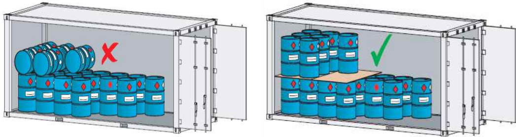
『직립 형태로 적재』
