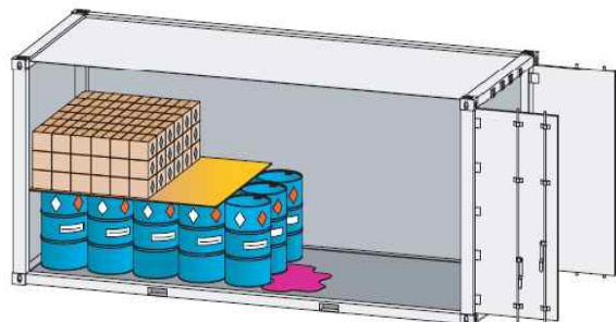
『하중에 따른 올바른 상하 적재위치』
