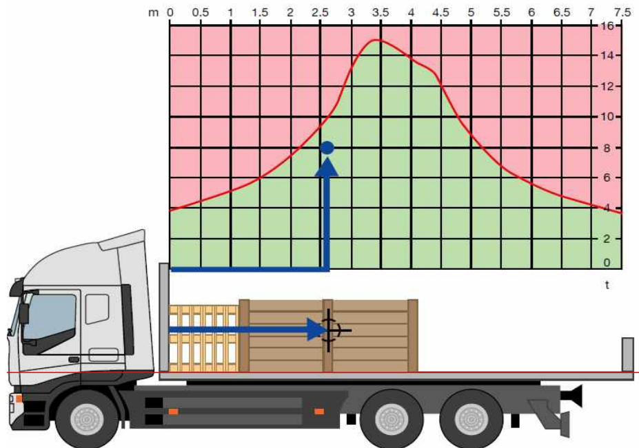
트럭에 대한 적재 배분표(load distribution diagram)의 예시
