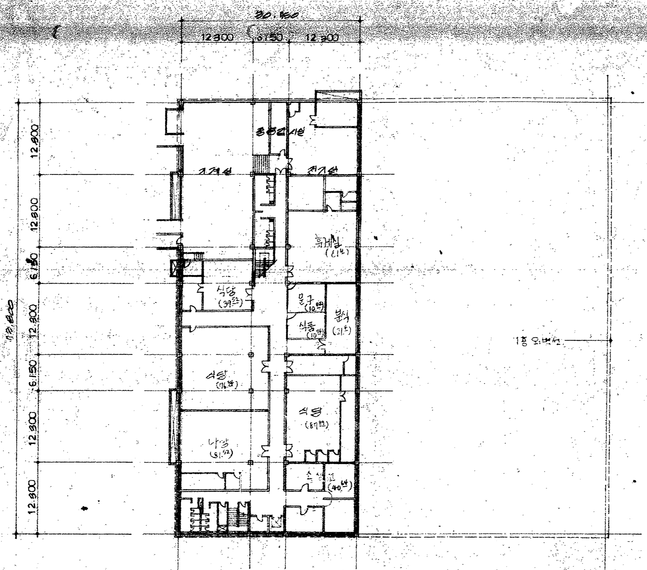
1 지하층 평면도 (원형 계획) SCALE 1/400
