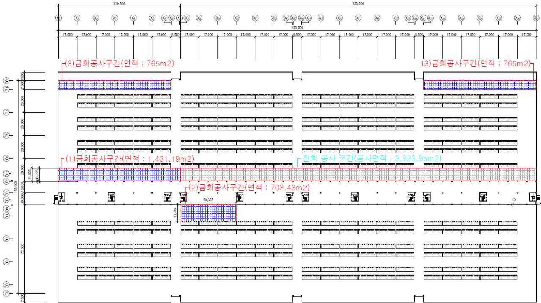
[청과물시장동 옥상 바닥 평면도]
