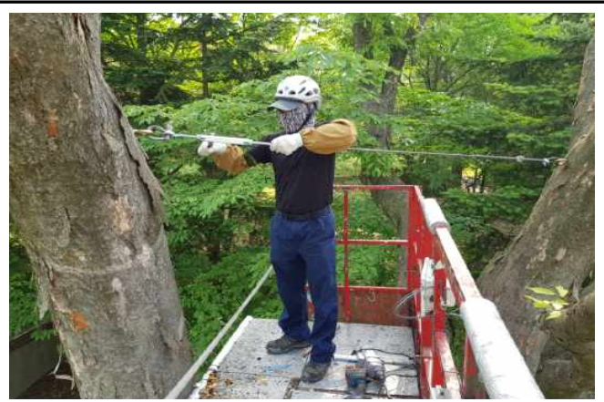
브레싱 설치(서12-10 느티나무)
