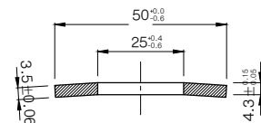
접시 스프링 와샤 S=1:1
