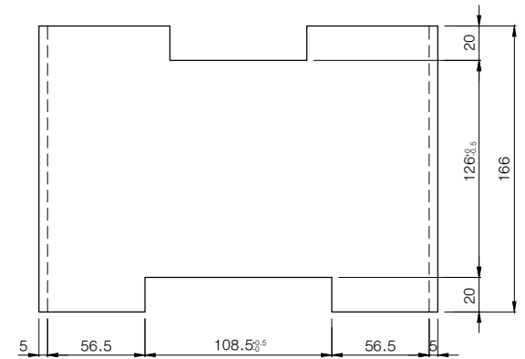
레일 패드 S=1:2
