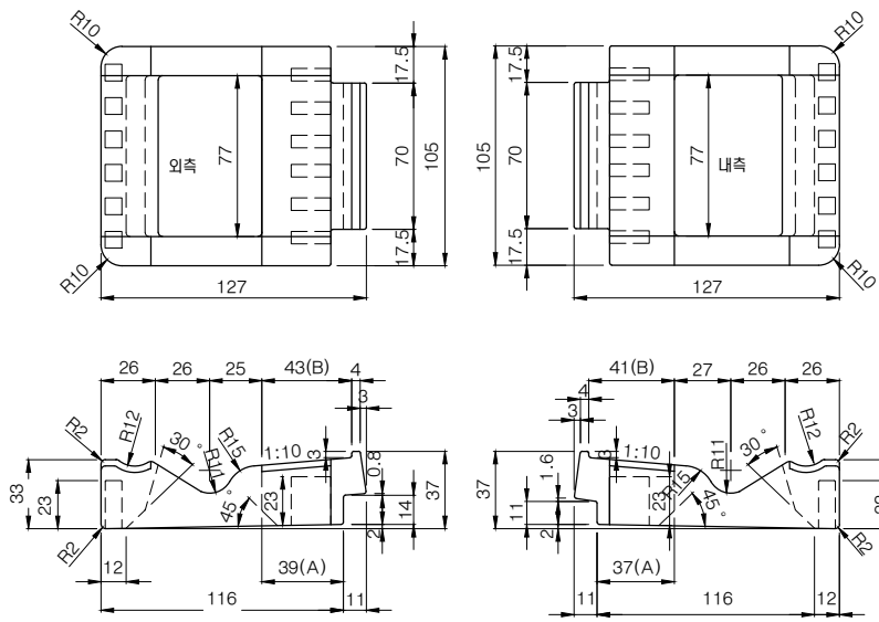
절연 블럭 S=1:2
