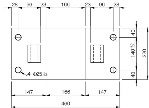
베이스플레이트 S=1:5
