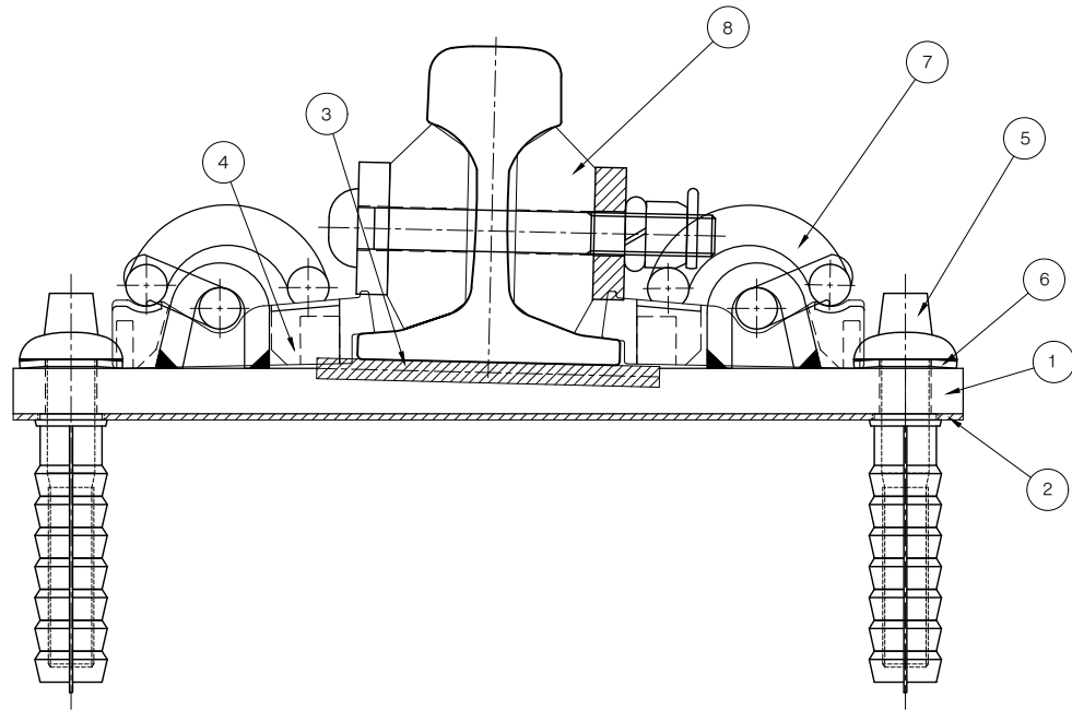
베이스플레이트 S=1:5
