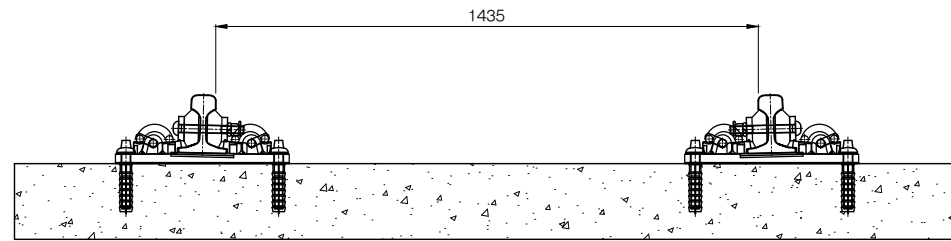
단면도 S=1:10
