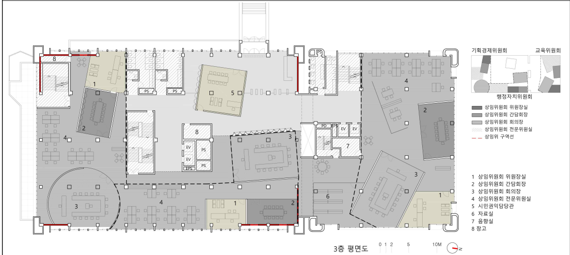
▲ 3층 평면도
