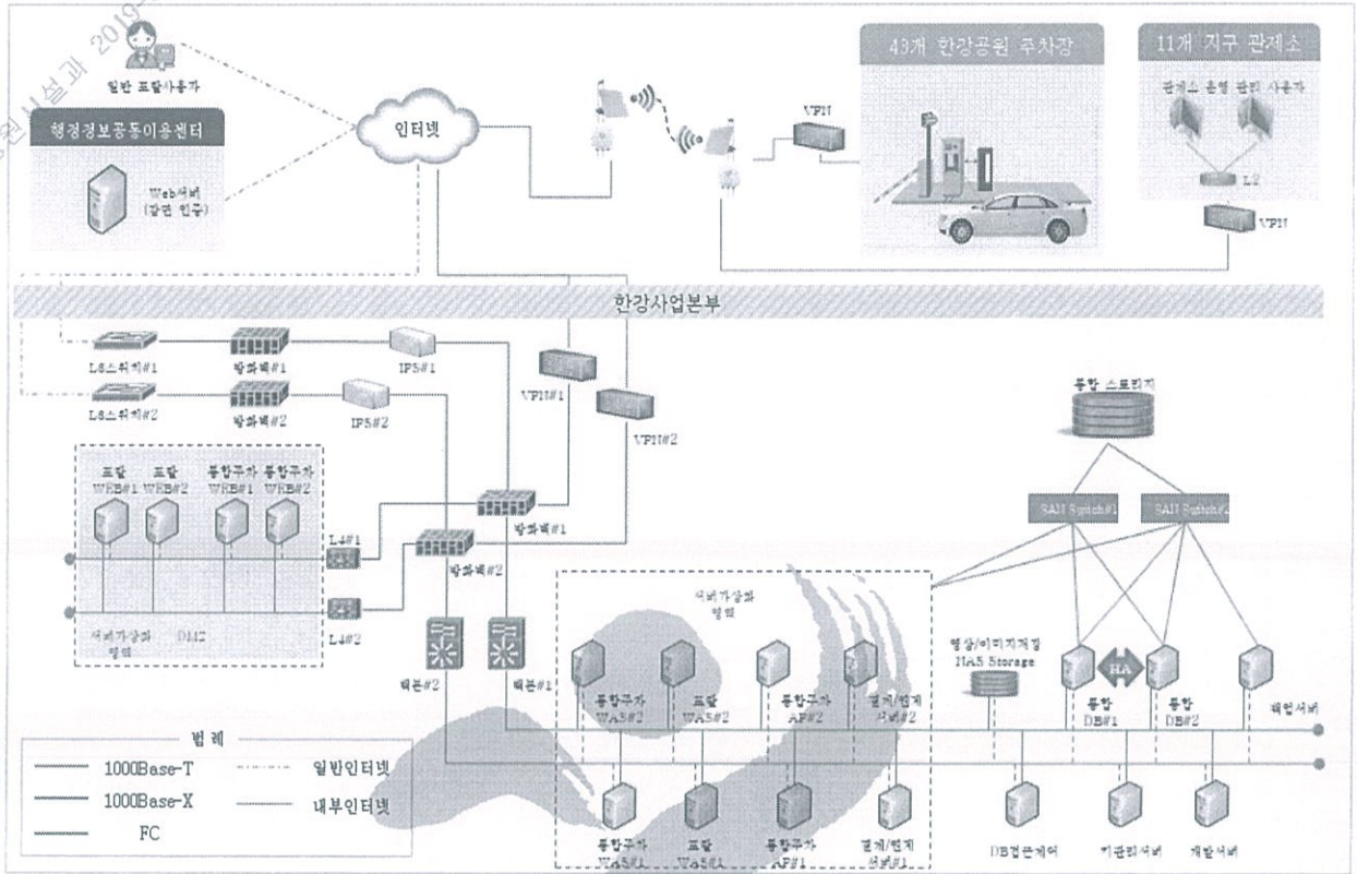
그림 1 목표시스템 HW 및 네트워크 구성도
