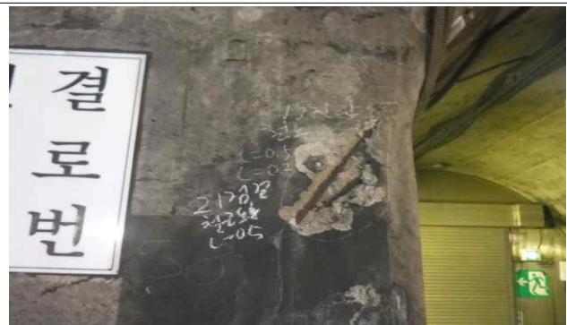
철근노출
