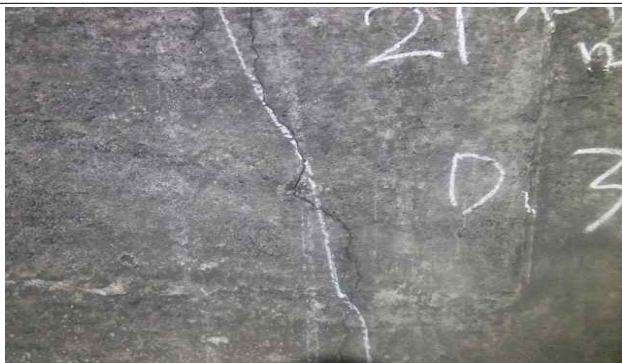
콘크리트 균열(0.3mm이상)
