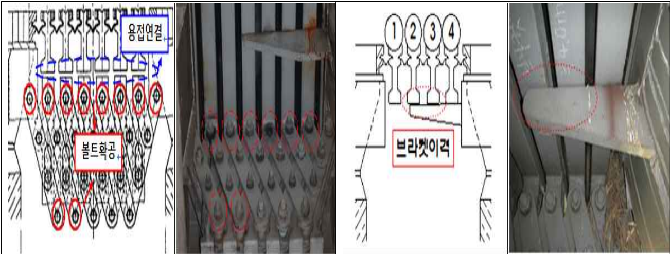
행거못치 모식도 및 전경(충격을 발생 및 볼트확공, 탈락) ❌
