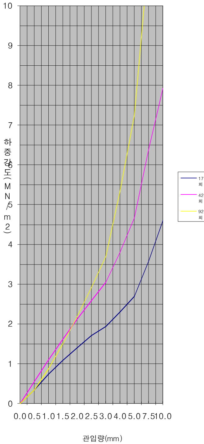
하중강도-관입량곡선
