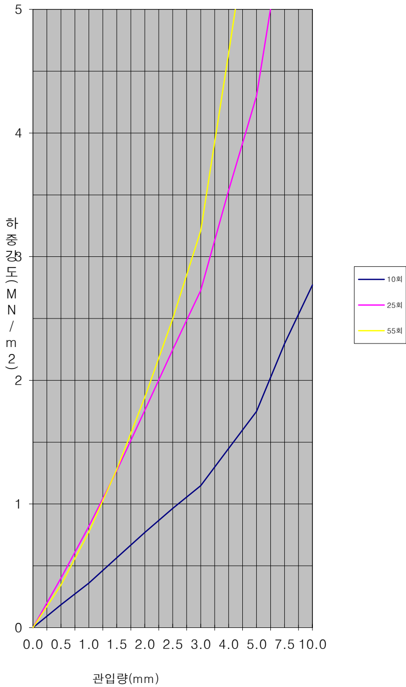
하중강도-관입량곡선
