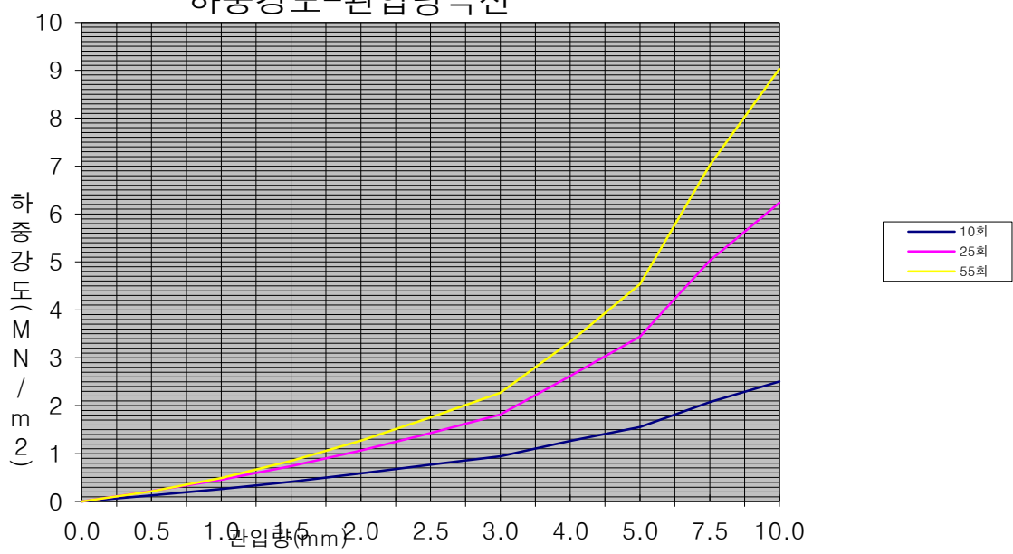
하중강도-관입량곡선
