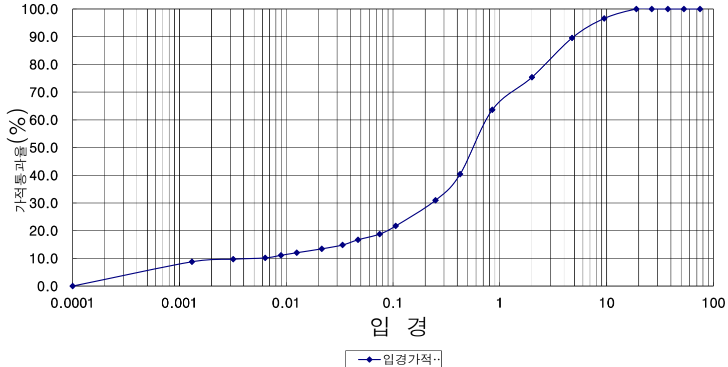
입경가적곡선
