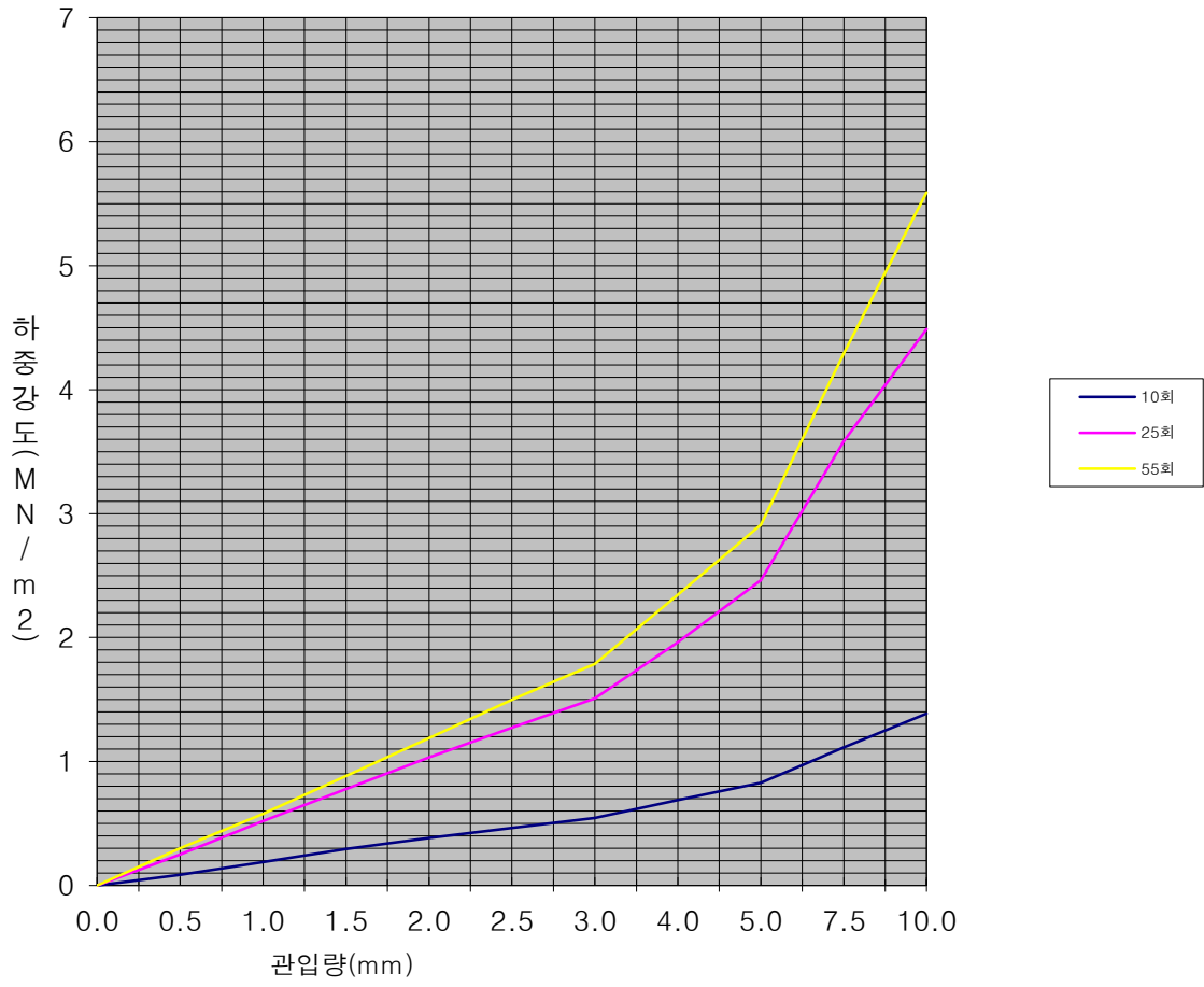
하중강도-관입량곡선
