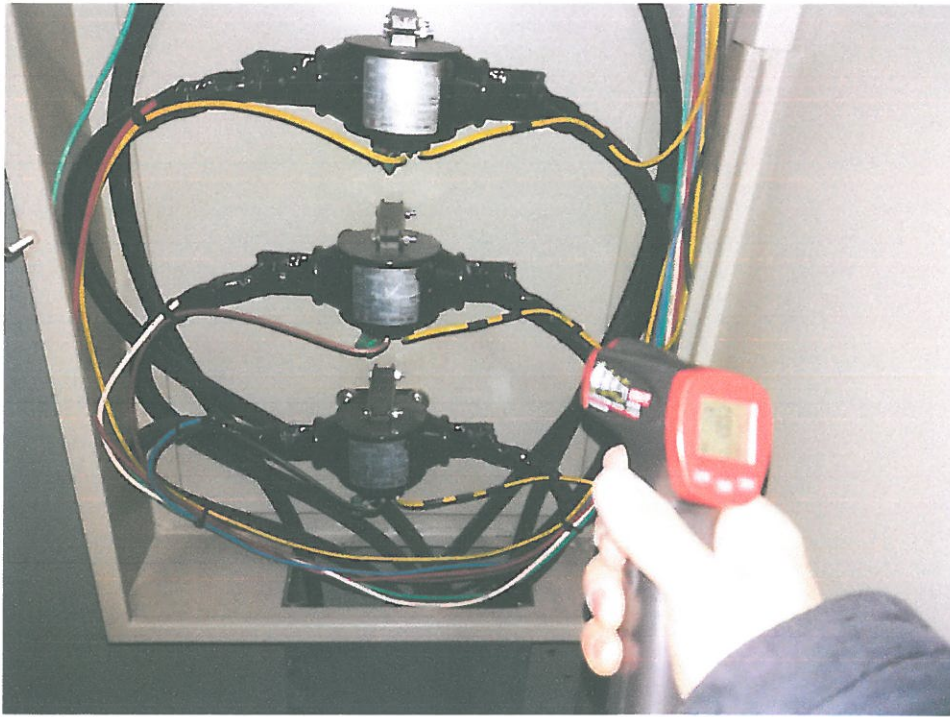
변류기 발열상태 점검(무지개터널)
