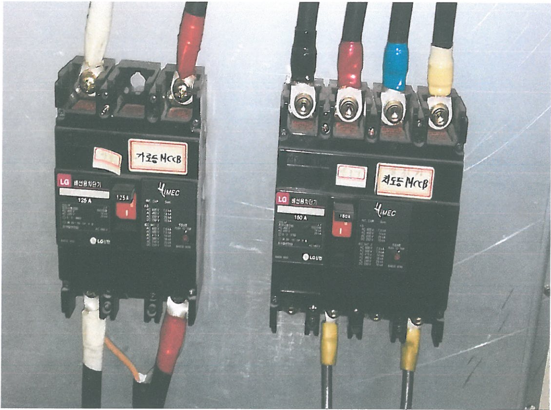
개폐기 선로 점검(동일로지하차도)
