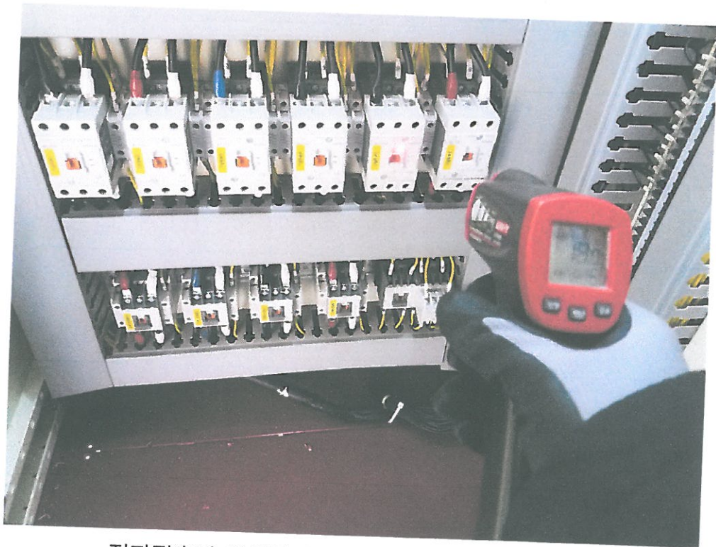
전자접촉기 발열상태 측정 및 점검(성동지하차도)
