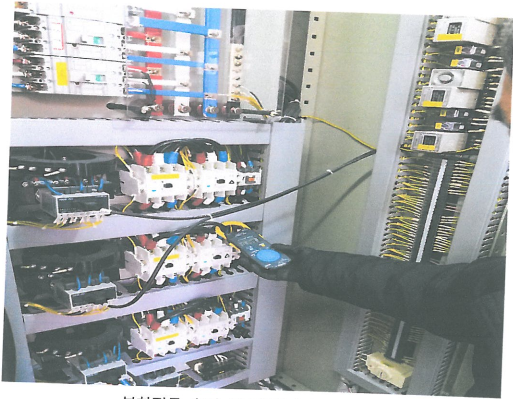
부하전류 측정 및 점검(마장지하차도)
