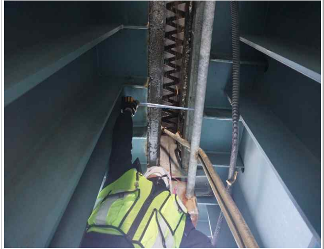
신축이음장치 유간 측정
