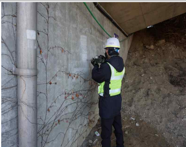
반발경도시험
