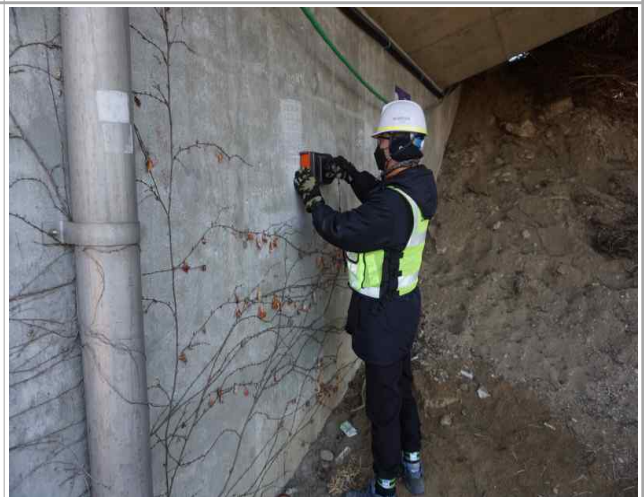
철근탐사시험
