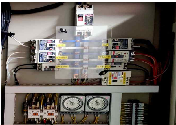
뚝섬벽천분수- 분전반 내부 M/G 상태확인
