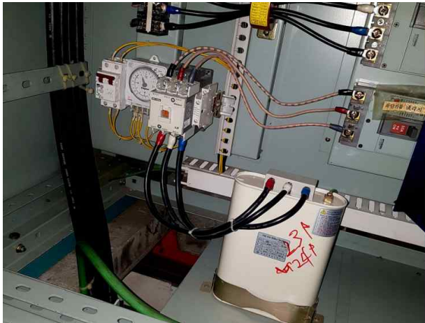
뚝섬벽천분수- 콘덴서 M/G 상태확인
