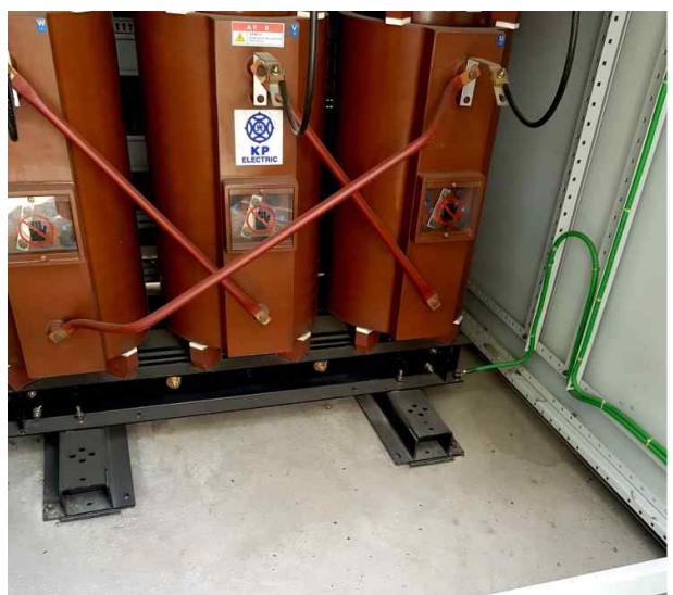
변압기반 빗물 유입상태 확인
