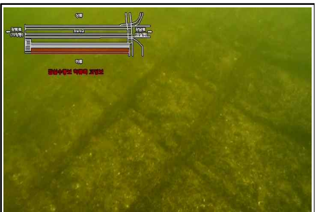
고정보 하류 STA.360m 철근노출
