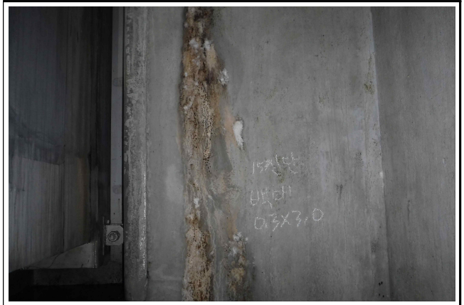
남단어도 기계실 벽체 누수 및 백태
