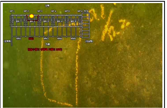
가동보 상류 MW2-2 표면침식
