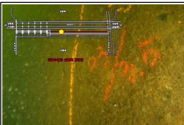
고정보 상류 STA.128m 균열(Cw=0.3mm, L=3.5m)
