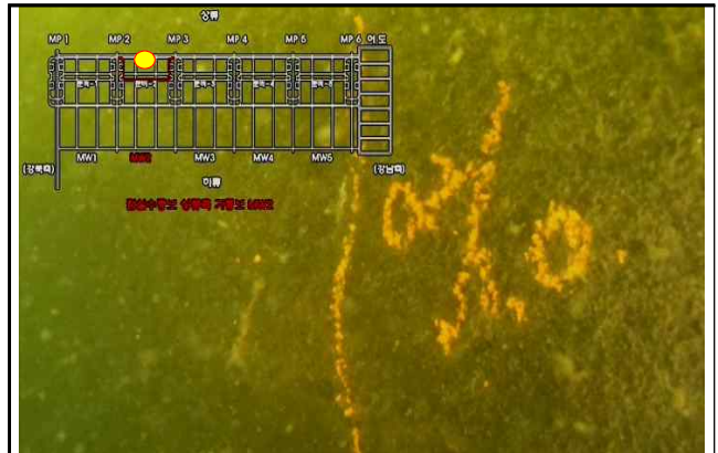
가동보 상류 MW2-2, 균열(Cw=0.2mm, L=1.0m)
