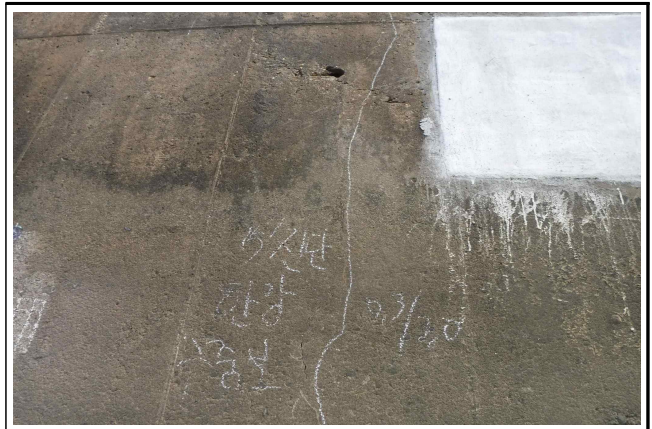
좌안옹벽 STA.088m 수직균열(Cw=0.4mm)
