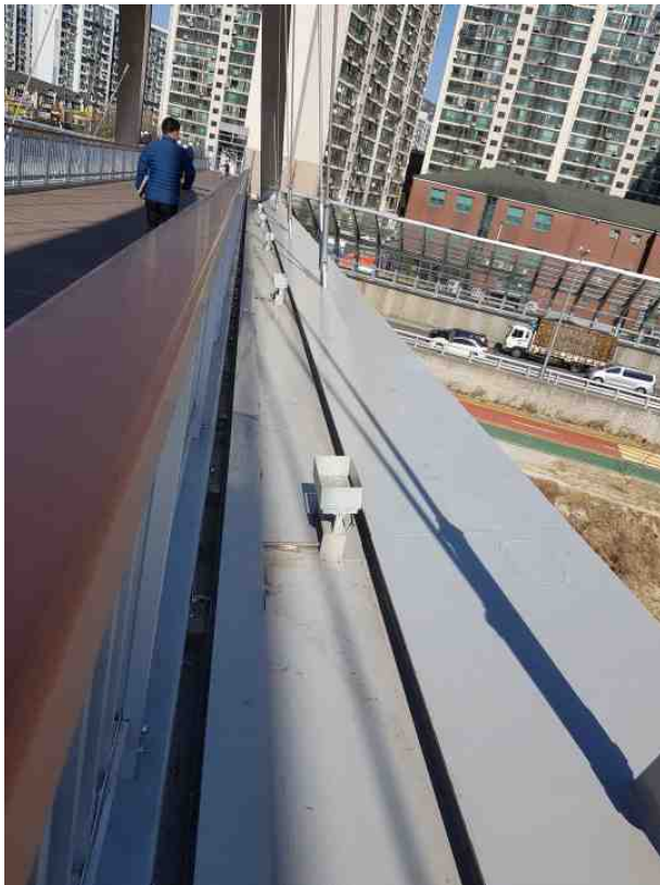
전선관 이탈(빗물유입우려)
