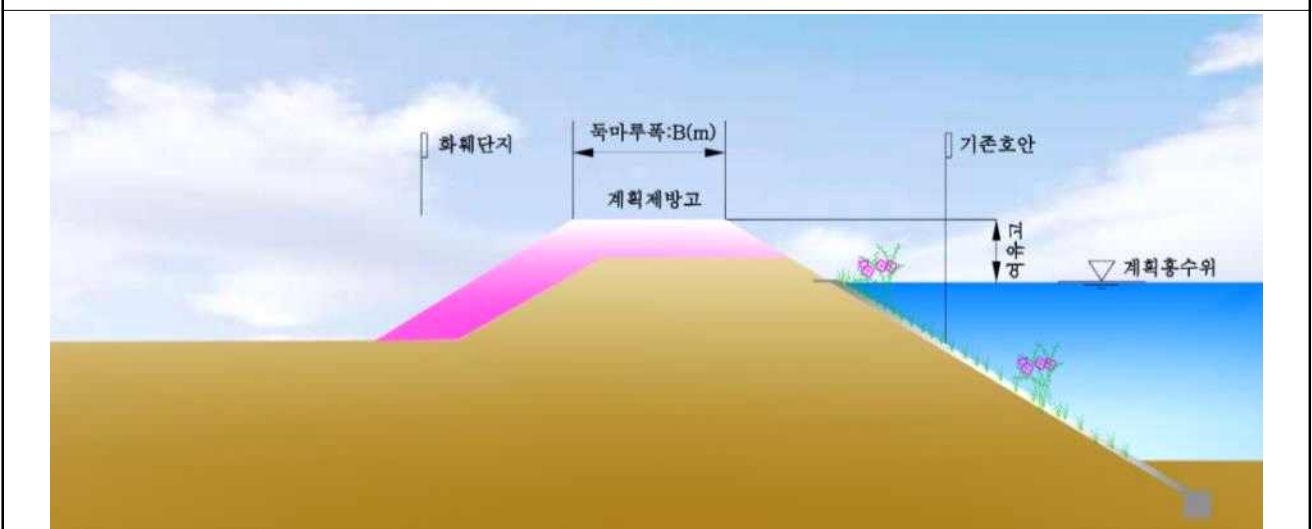
단면도
