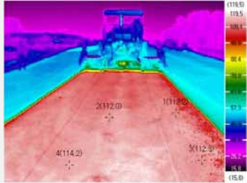
〈 아스팔트 혼합물의 균질한 포설면 유지 〉
