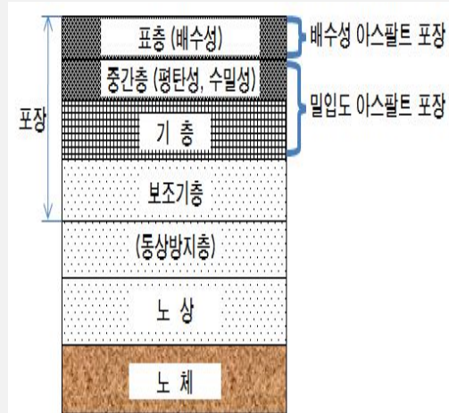
〈배수성 아스팔트 콘크리트 포장의 구성〉
