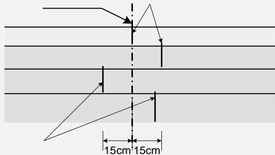
< 포장층 세로 시공이음부 (예) >
