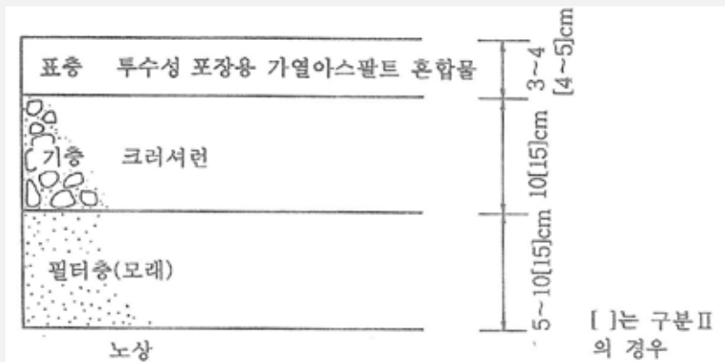
〈투수성 포장용 가열 아스팔트 혼합물에 의한 포장구성〉
