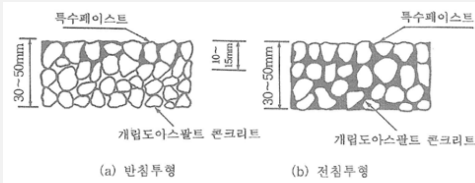
<반강성포장의 표준단면도>
