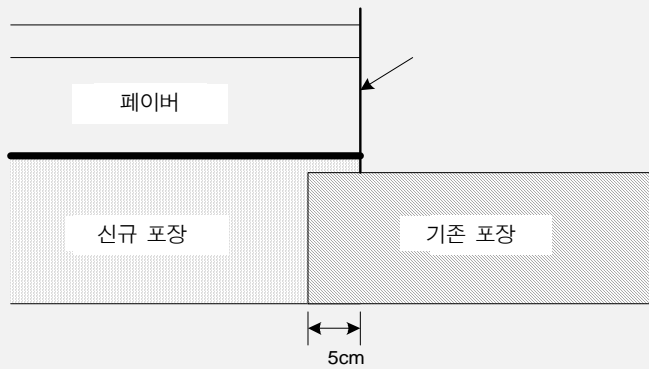
< 포설작업 시 세로 시공이음부의 겹침 >
