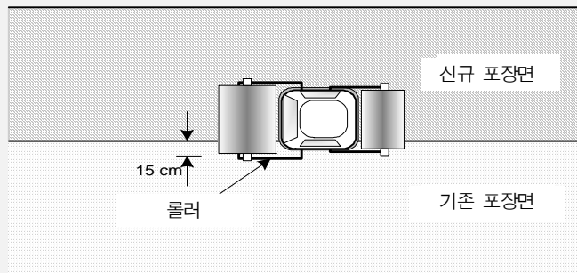
< 기존 포장과 신규 포장 세로 시공이음부 시공 >
