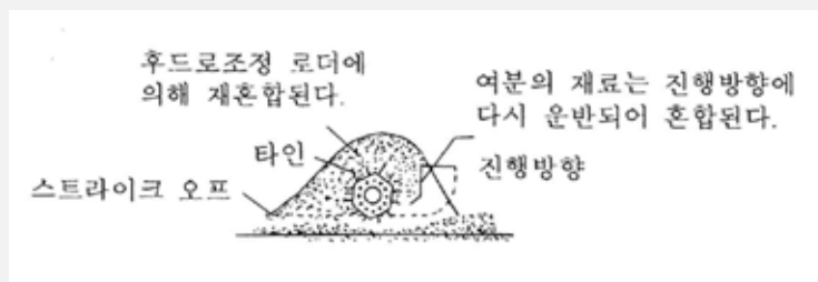
〈횡축식 로드스테빌라이저의 혼합기구〉
