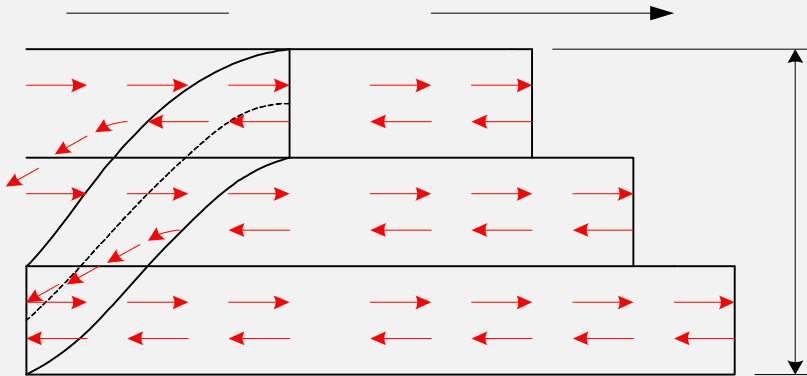
< 롤러에 의한 다짐 방법 (예) >
