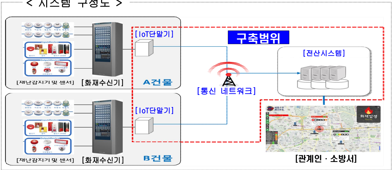
< 시스템 구성도 >
