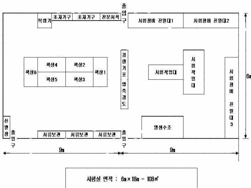
시험실 배치 평면도
