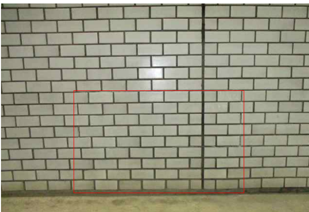
신길지하차도 전경 (우측벽체 타일들뜸)
