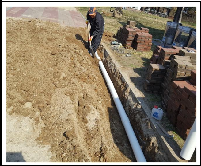
9. 통기관 배관
