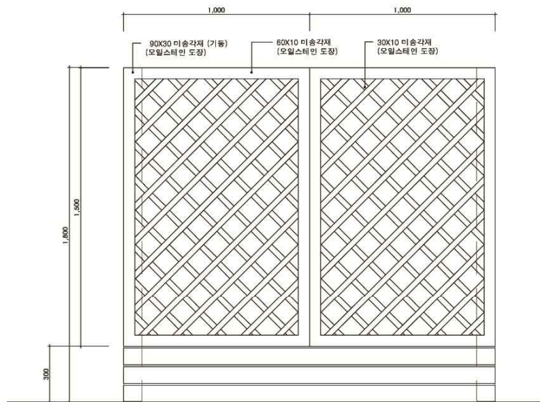
1 목재 플랜터 단면도 축척 : A1=1/10 A3=1/20
