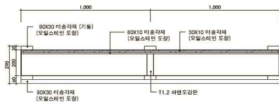
1 목재 플랜터 단면도 축척 : A1=1/10 A3=1/20
