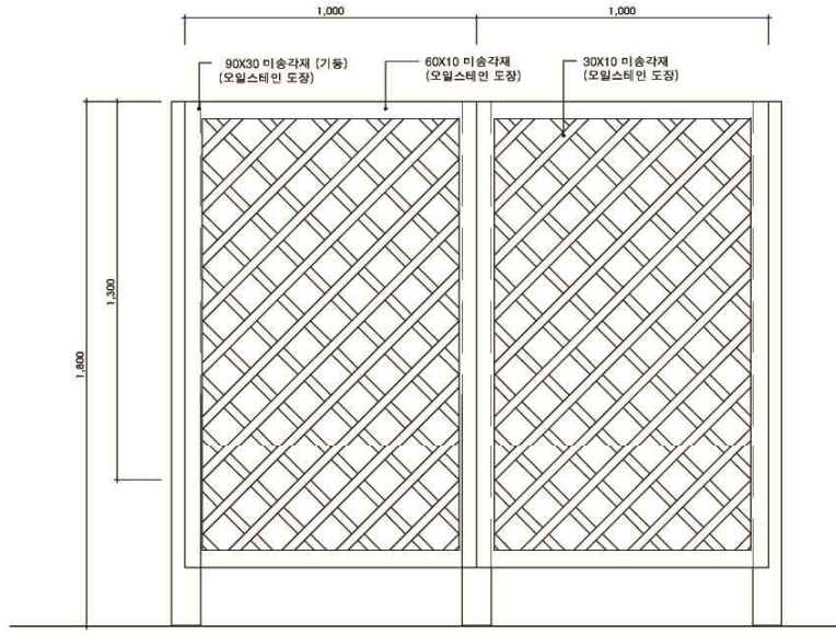
2 목재트렐리스 정면도 축척 : A1=1/10 A3=1/20
