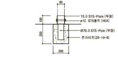
4 기초상세도 축척 : A1=1/10 A3=1/20
