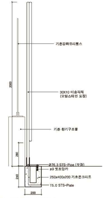
3 목재트렐리스 측면도 축척 : A1=1/10 A3=1/20
