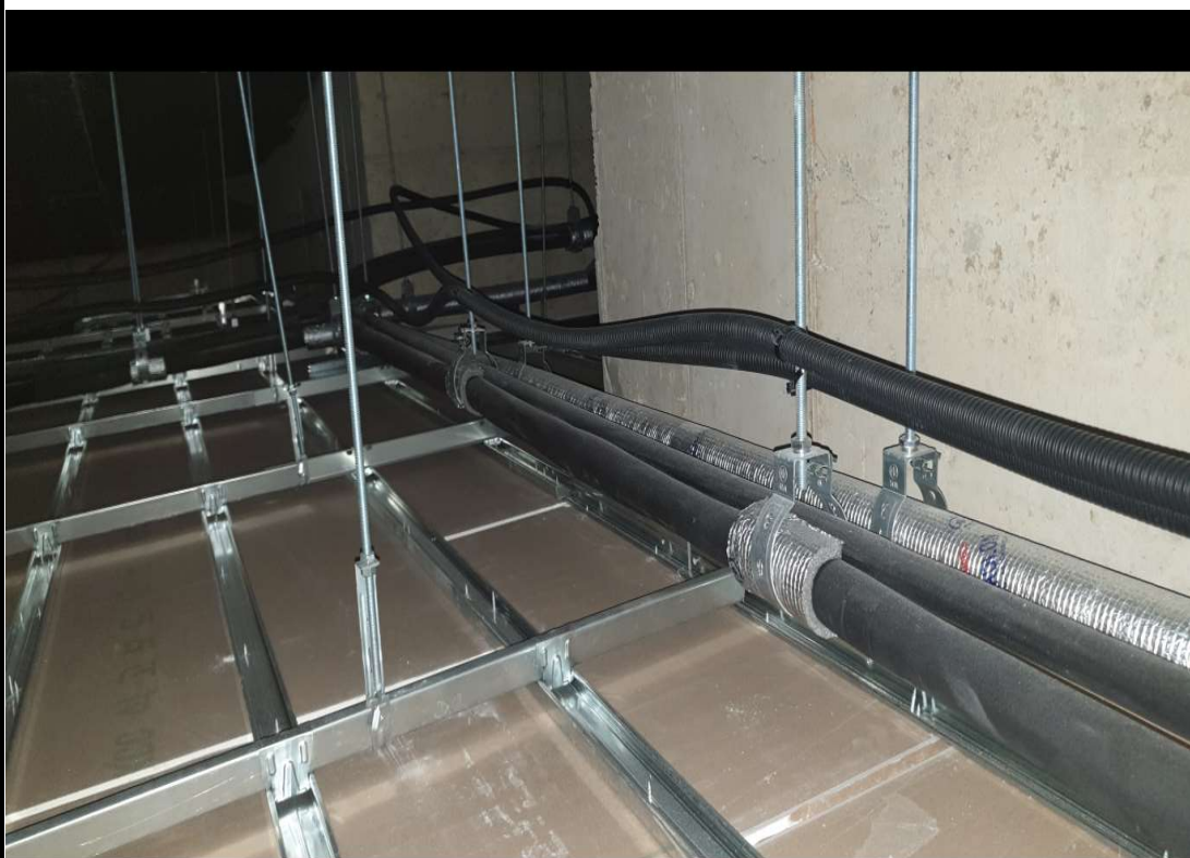
배관작업-2
