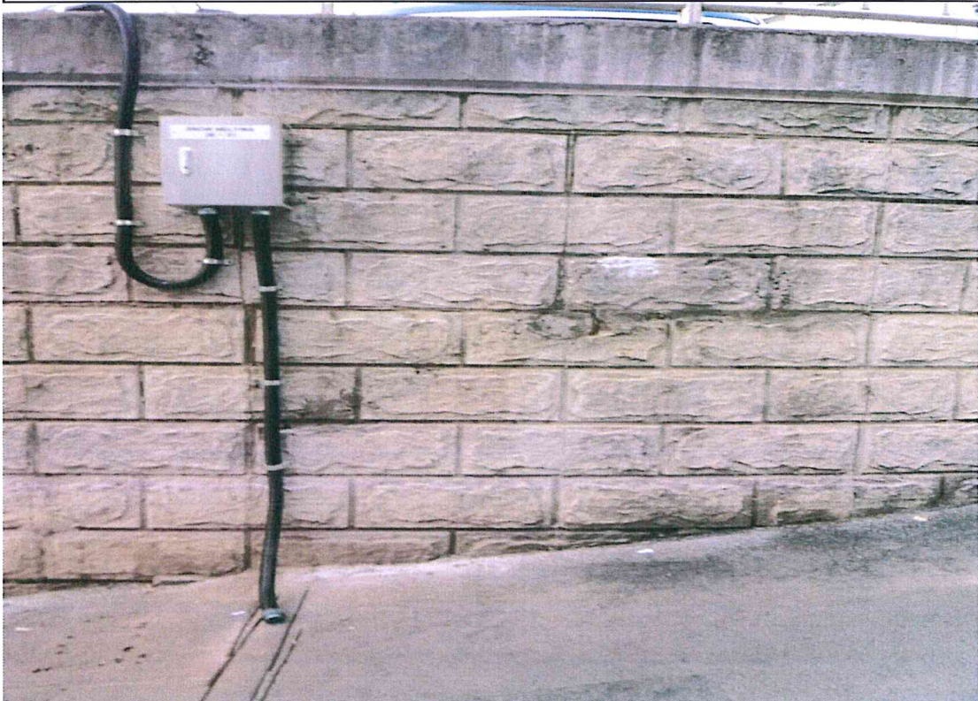
분전함설치 후
