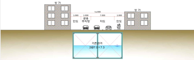
카페골목 구간 횡단면도
