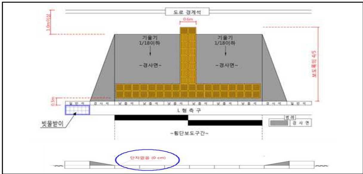
▶ 횡단보도 턱낮춤 기준
