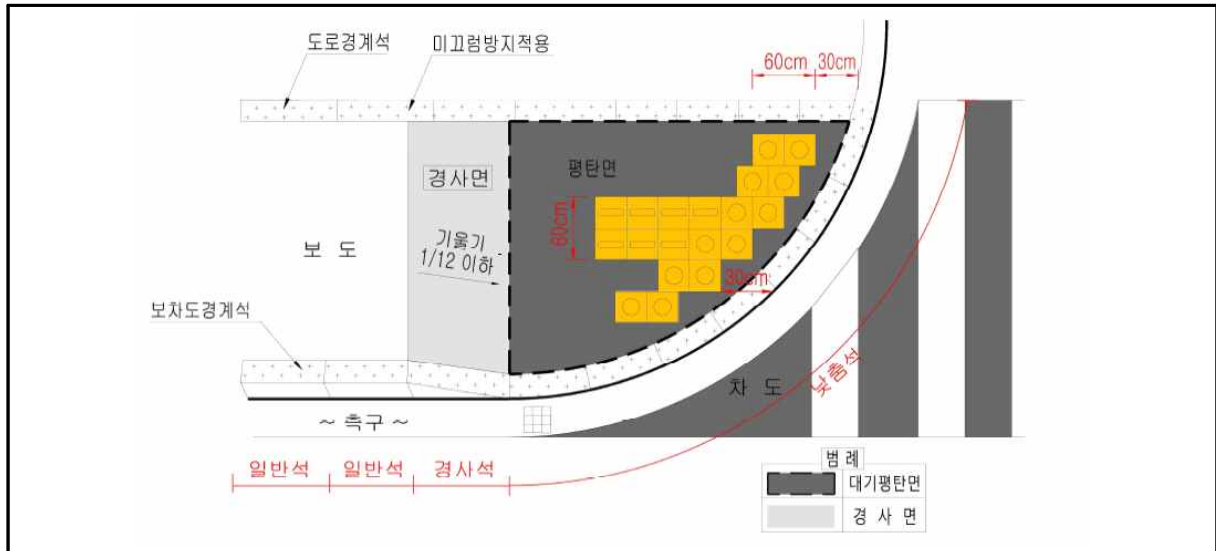
▶ 도로곡선부 턱낮춤 기준
