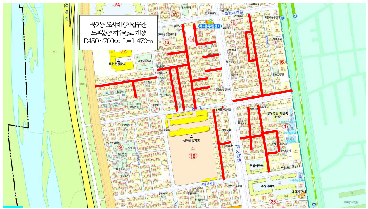
위 치 도 (노후 하수관로 정비)
