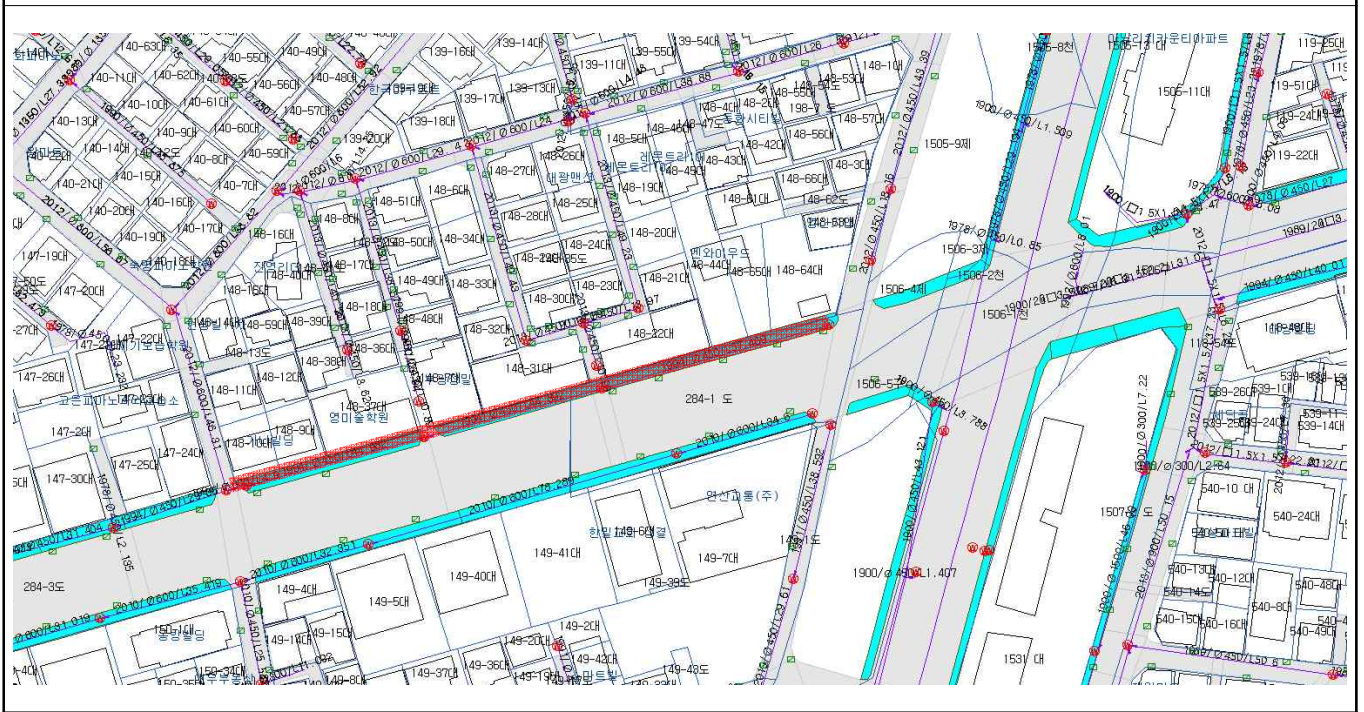
하수관망도(면목동 148-10~148-64)
