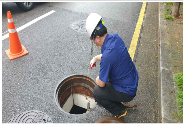
전송반 점검(천호증압장)
