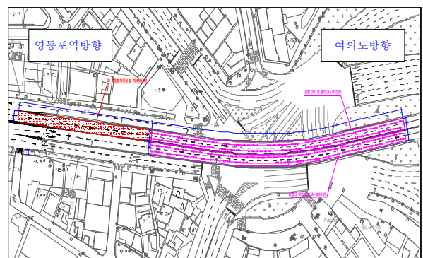
미끄럼방지시설 설치계획도
