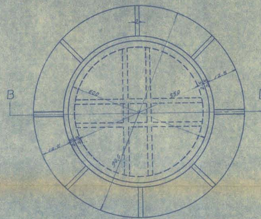
人孔蓋詳細 S = \frac{1}{10}
