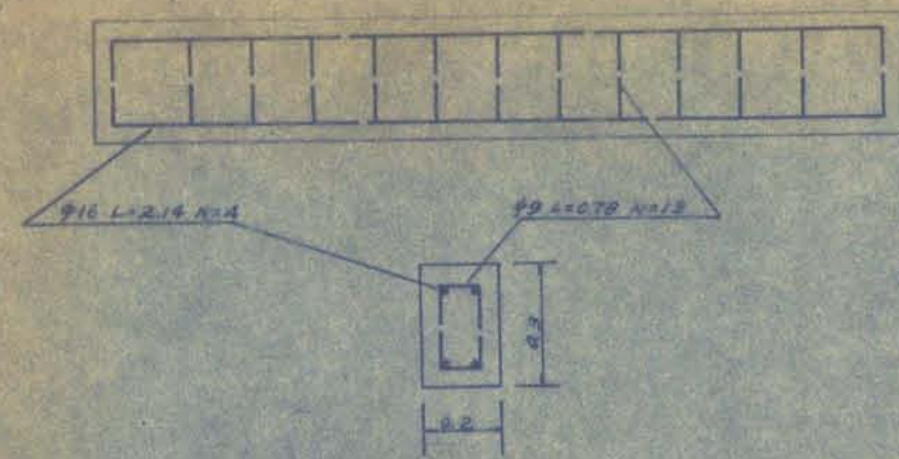
부식詳細 S = \frac{1}{20}
