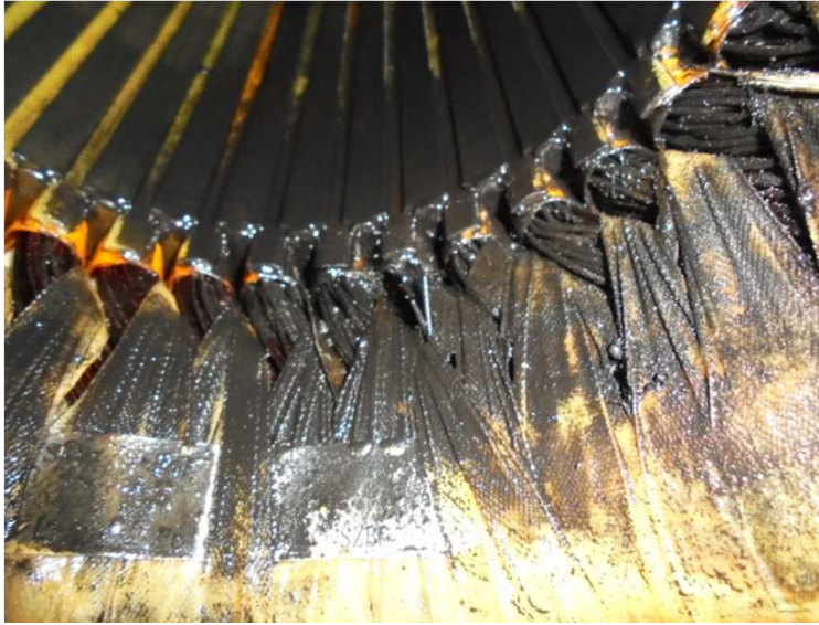
모타 권선 교체전
