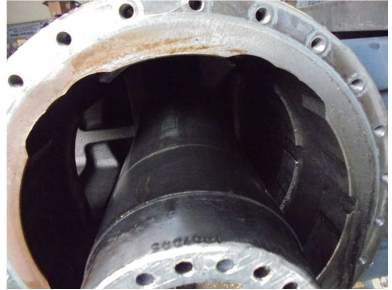
압축기 분해
