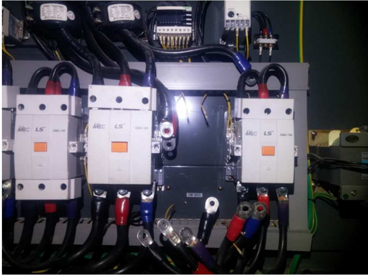
마그네트 교체전
