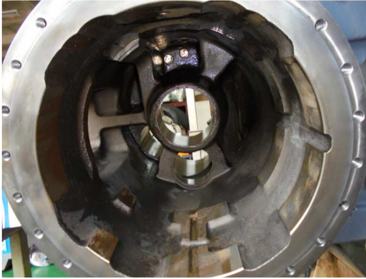
압축기 분해
