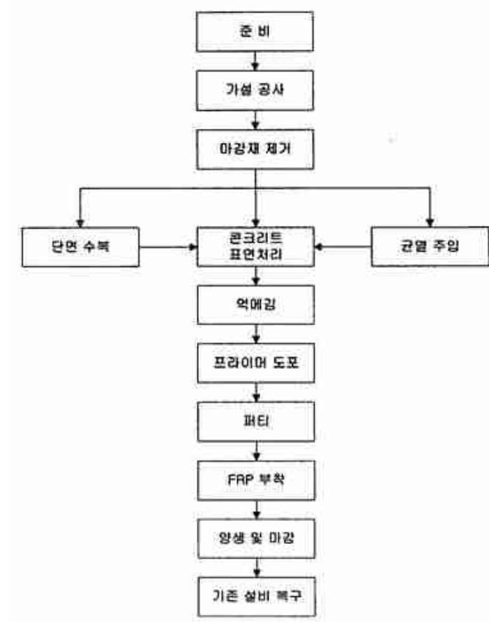
<섬유보강공법 시공순서>
