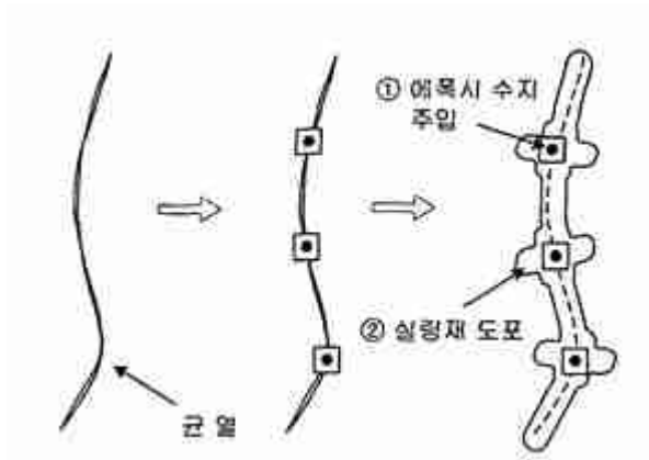
<그림 1.3> 수동식 주입공법
