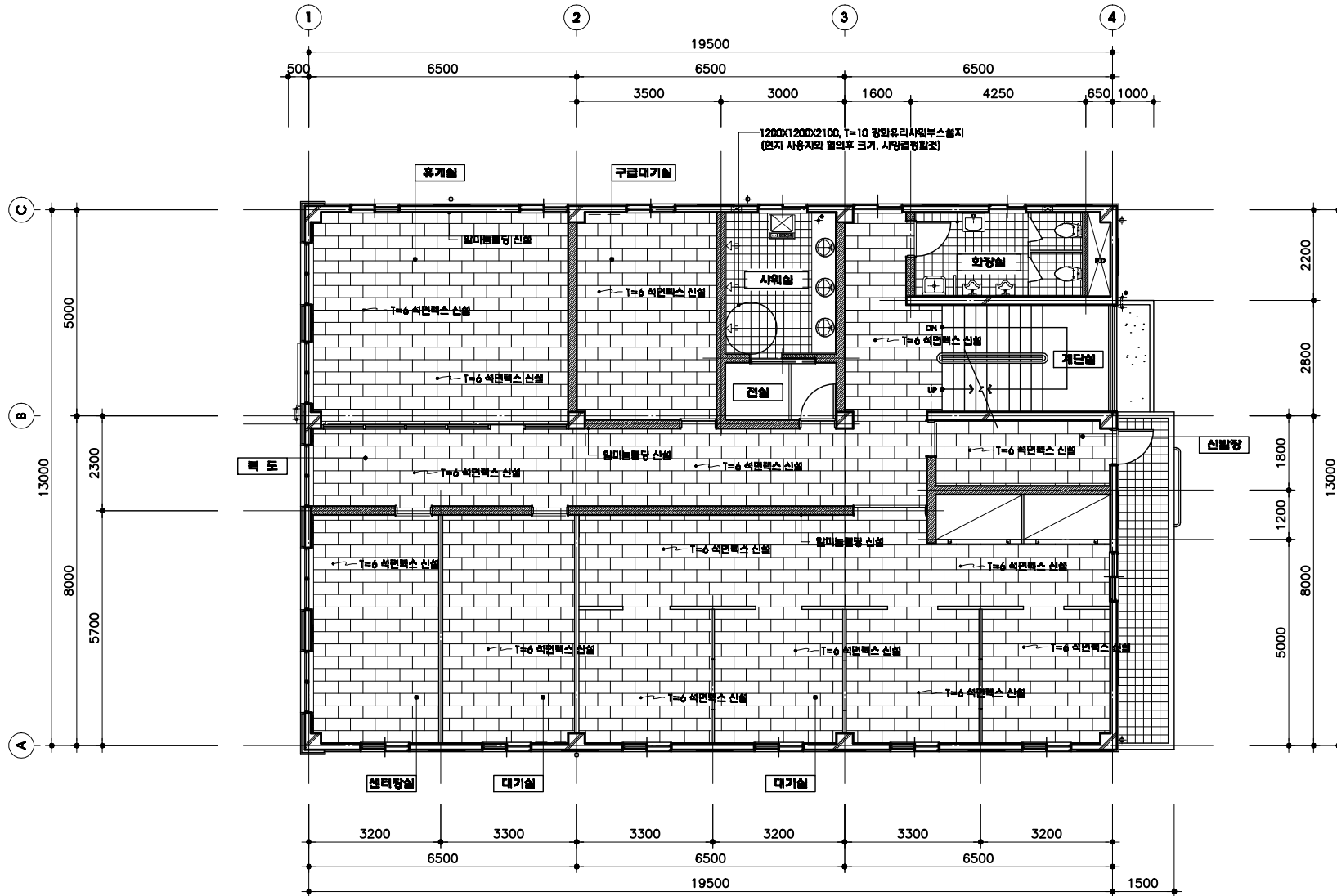
⊙ 2층 천장 평면도 [신설] (영동119 안전센터) SCALE: 1/80(A1) SCALE: 1/100(A3)
