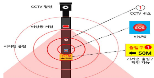
복합형 음향시설 설계안(스피커, CCTV, 비상벨 등)
